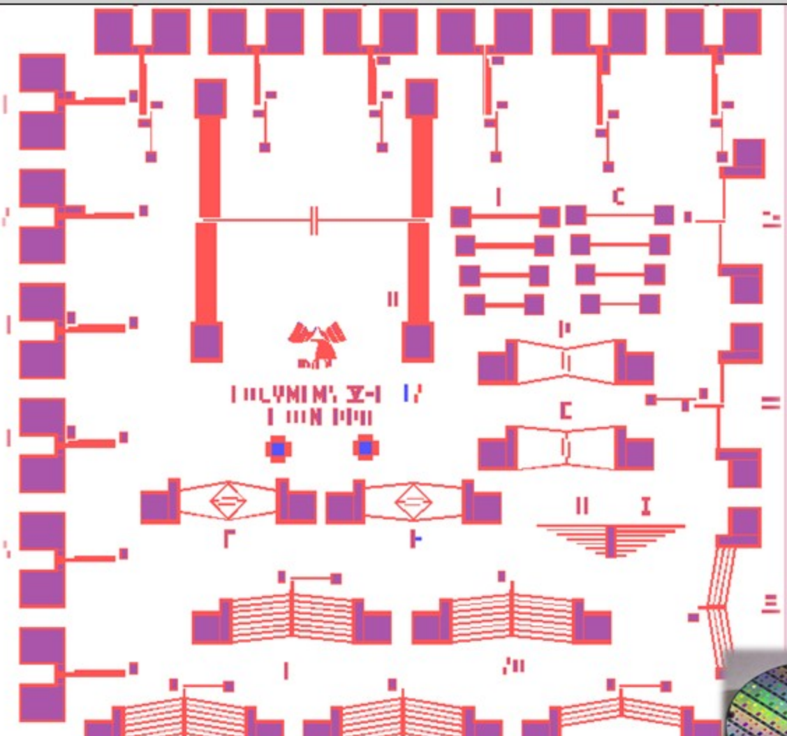
Tecnología PolyMEMS INAOE
